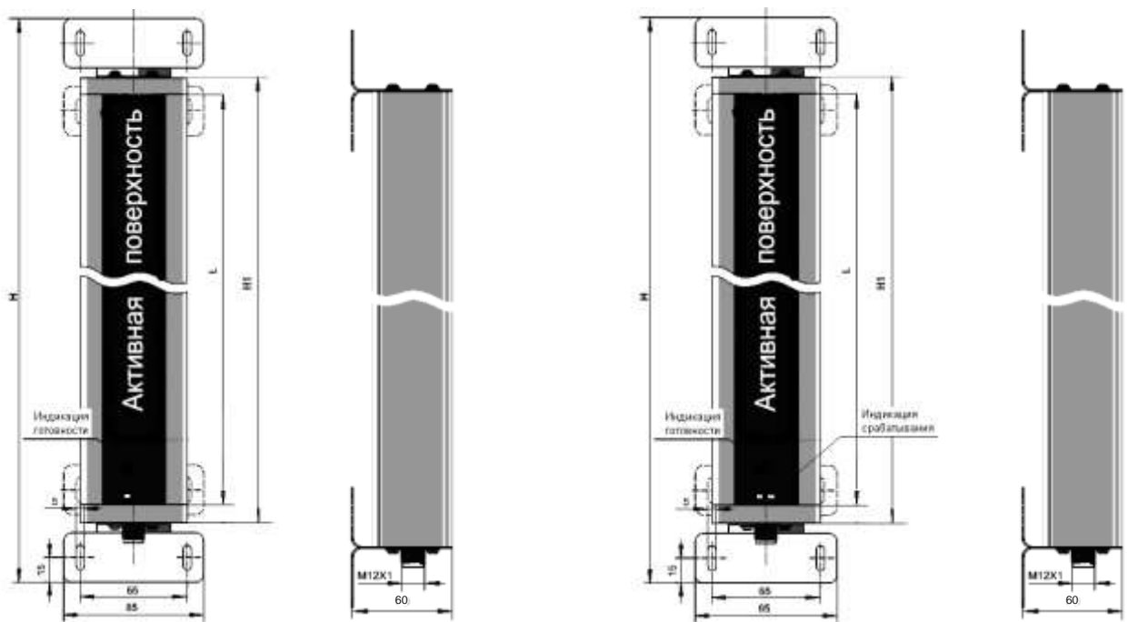
ВБО-Э10/20/40 излучатель
