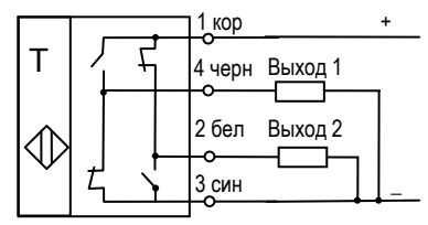
Рис. 4. Приемник Выход 1 – PNP, НО Выход 2 – PNP, НЗ
